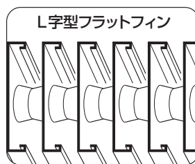
ラジエーター 水平断面図
