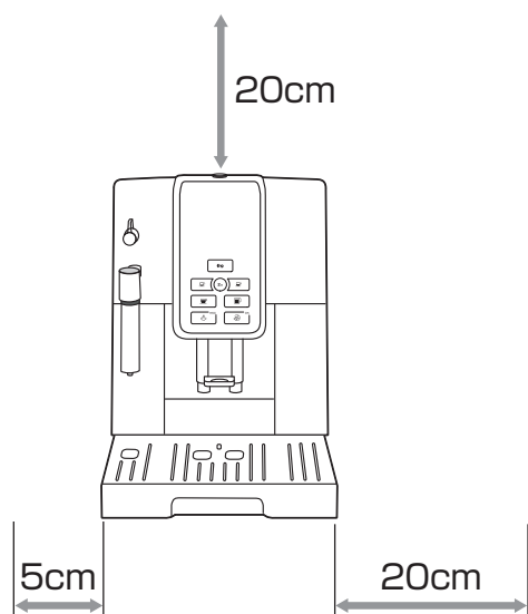
〔本体正面〕
