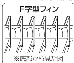
ラジエーター水平断面図
