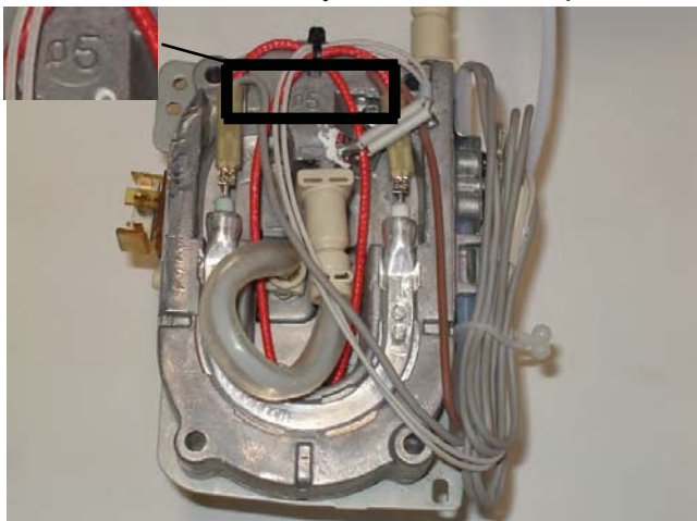
Foto 2: 5513227901 (Caldaia Ø5 X 0.5)
